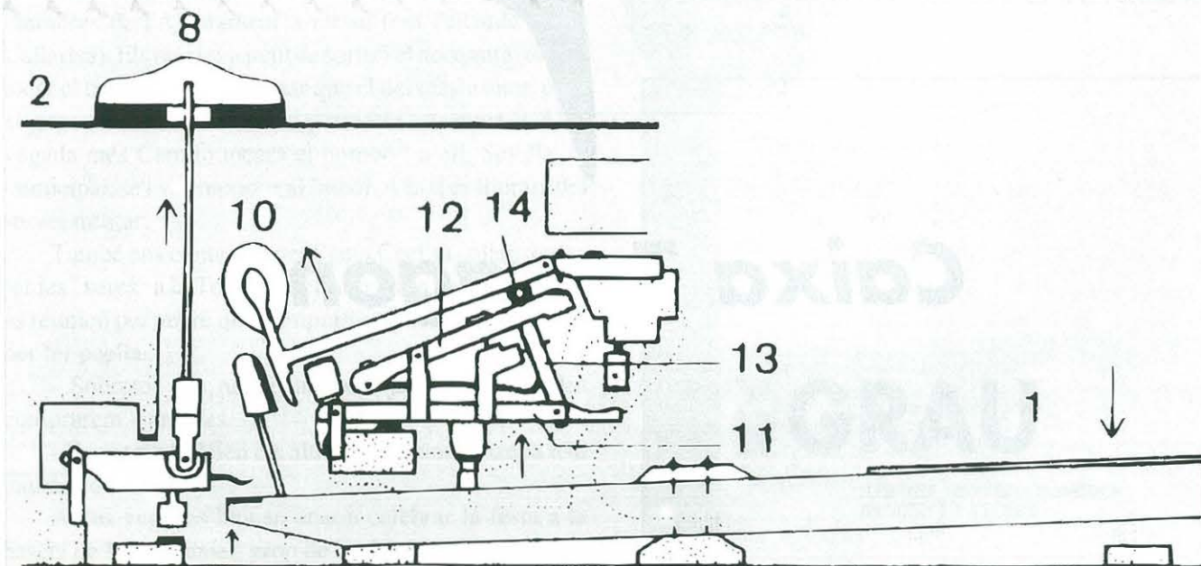
MECANISME D'UN PIANO
